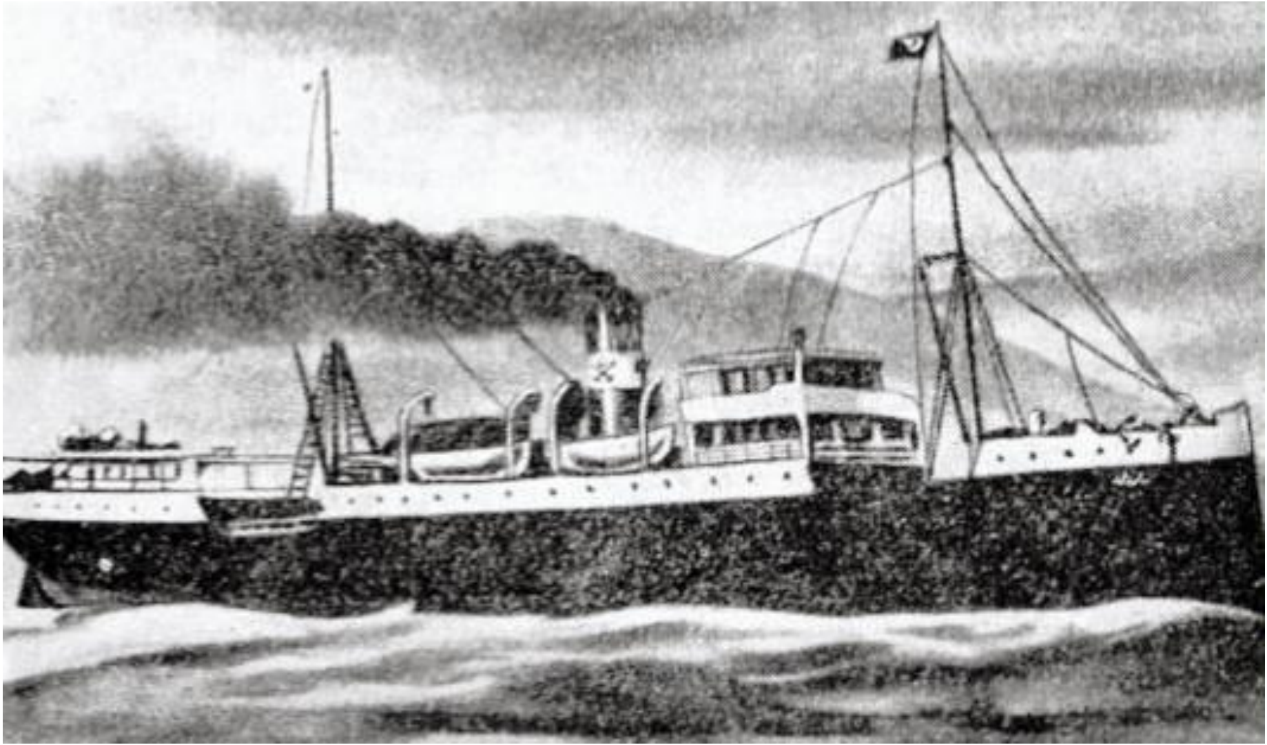
Bandırma Vapuru
