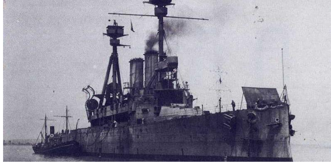
Agamemnon Zırhlısı
